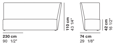
cod. 3521 / B_right element 230 H.110
